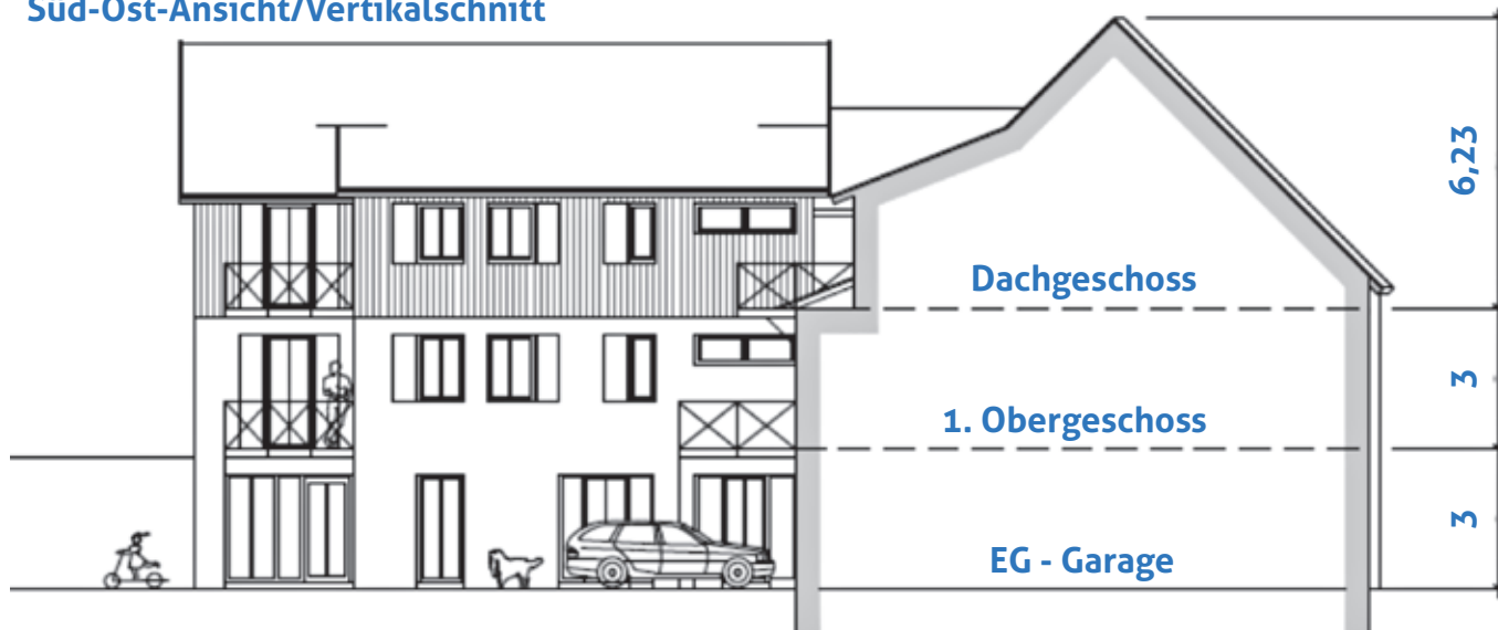
Süd-Ost-Ansicht/Vertikalschnitt
