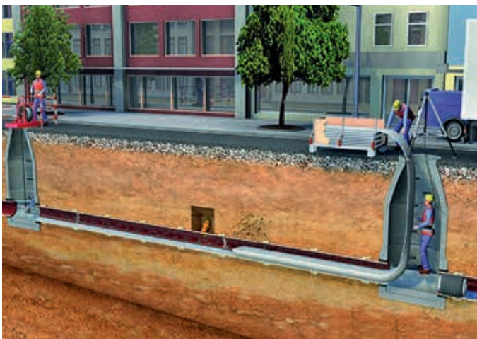
Systemzeichnung - Einzug des Liners Foto: Swietelsky-Faber
