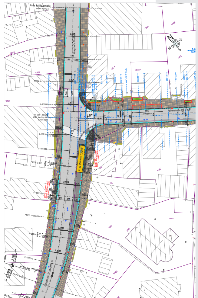
Umbauplan des Einmündungsbereichs NES in die NES 20 Quelle: Ingenieurbüro Stubenrauch
